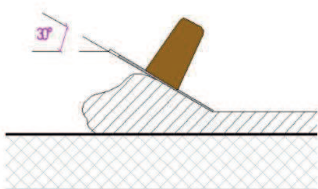
Espalhamento da argamassa colante com desempenadeira lado liso em um ângulo de aproximadamente 30^\circ
